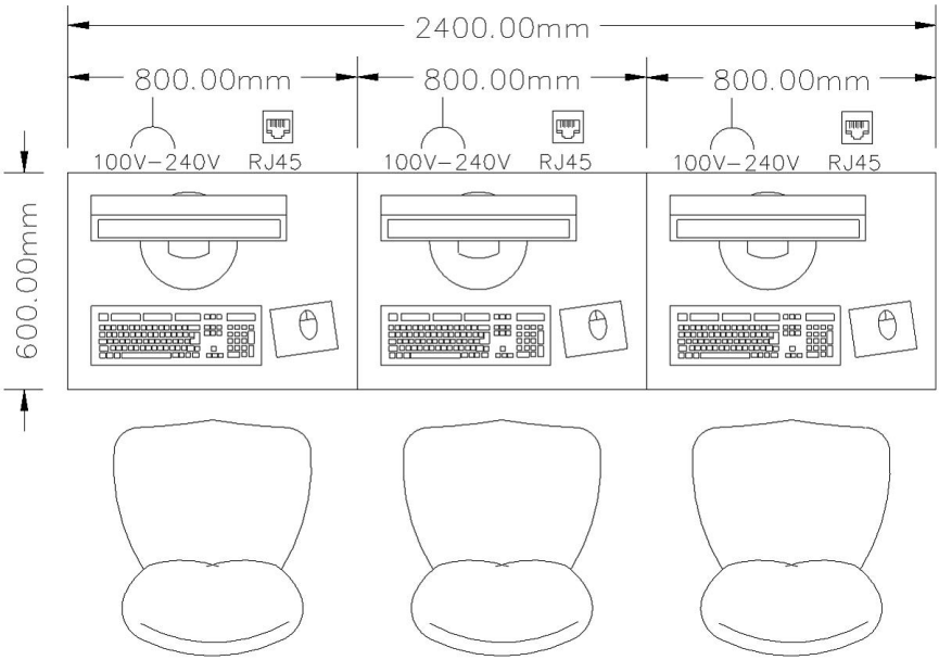
工位布局图
