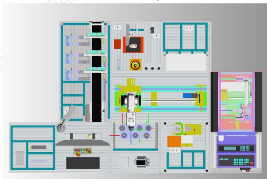
图 A-2 组装后俯视图
