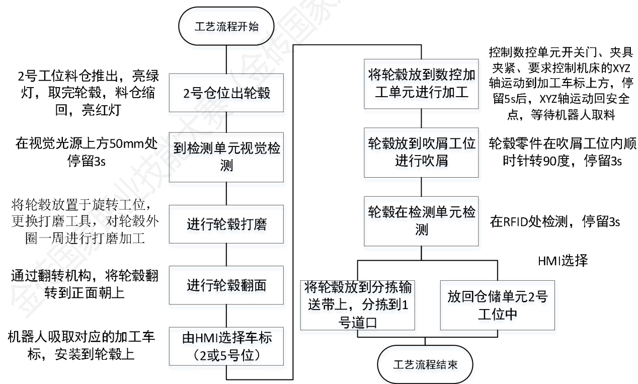
图 A-3 工艺流程图
