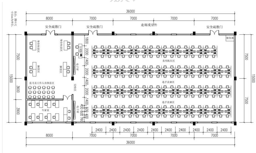
图 1 比赛区域和工作站布置图
