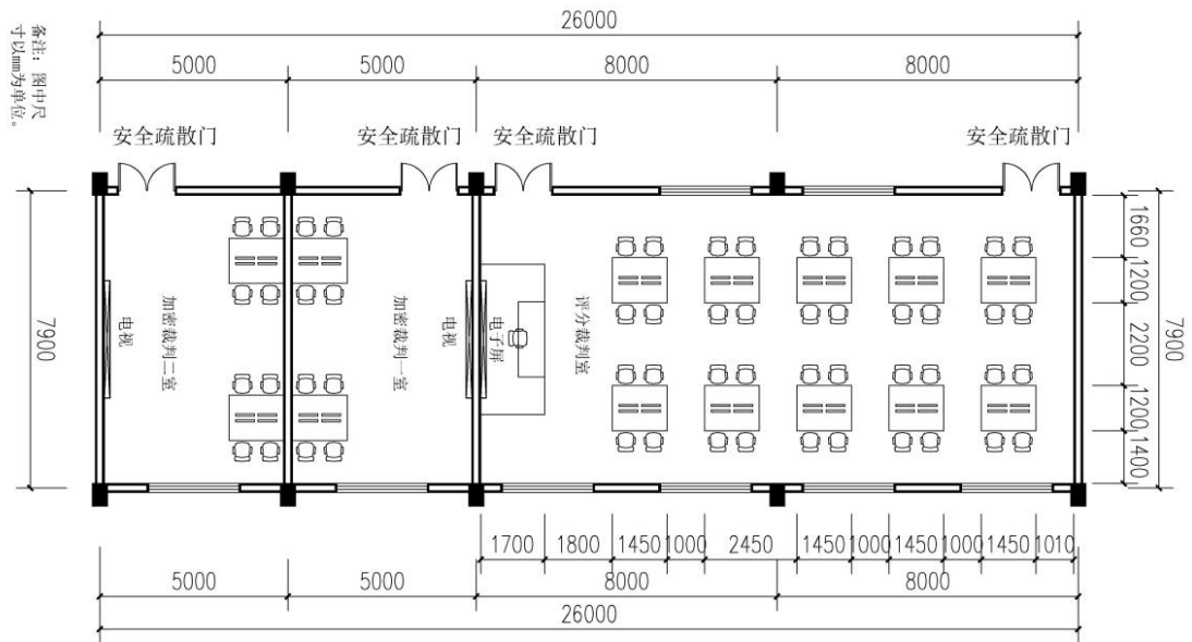
图2 评分裁判室和加密室布置图
